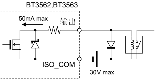
与继电器的连接
