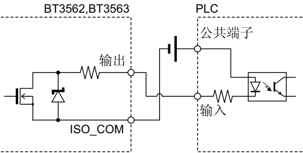
与 PLC 输入（负公共端子输出）的连接
