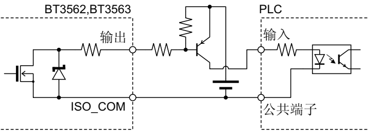
与 PLC 输入（正公共端子输出）的连接
