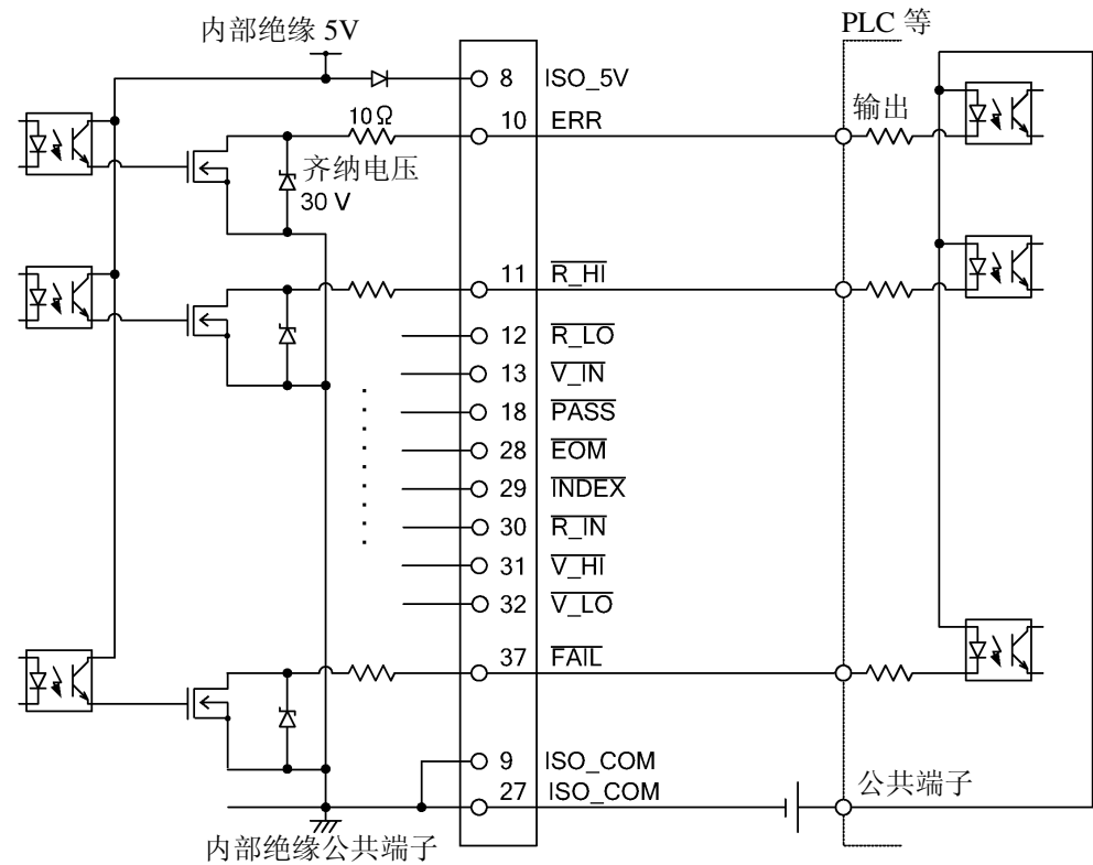
输出电路
