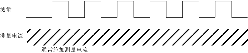
通常测量内部触发时的测量和电流施加 （测量电流脉冲输出功能 =OFF 时通常施加测量电流）
