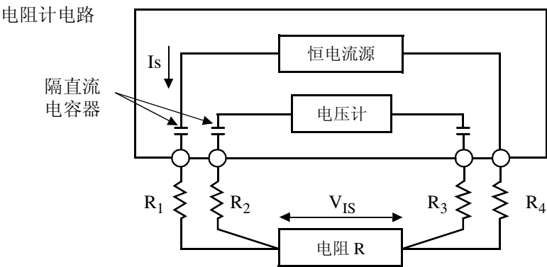
R_1 \sim R_2 : 测试线的电阻和接触部分的接触电阻
