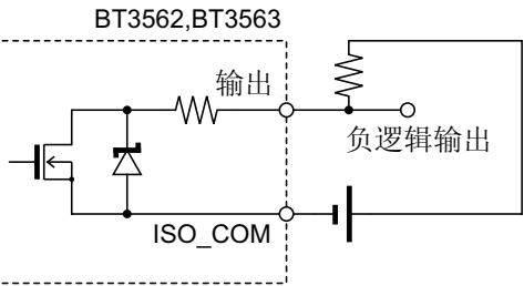
负逻辑输出
