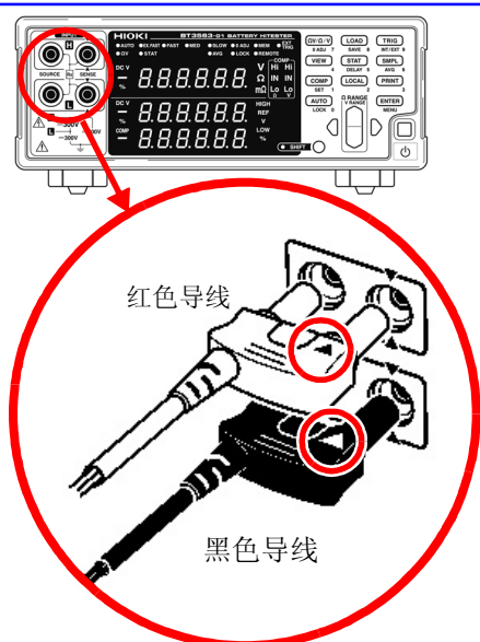
<例> L2107 夹型测试线（选件）
