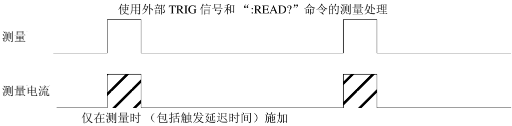
外部触发测量或连续测量 =OFF(:INIT:CONT OFF) 时的测量和电流施加
